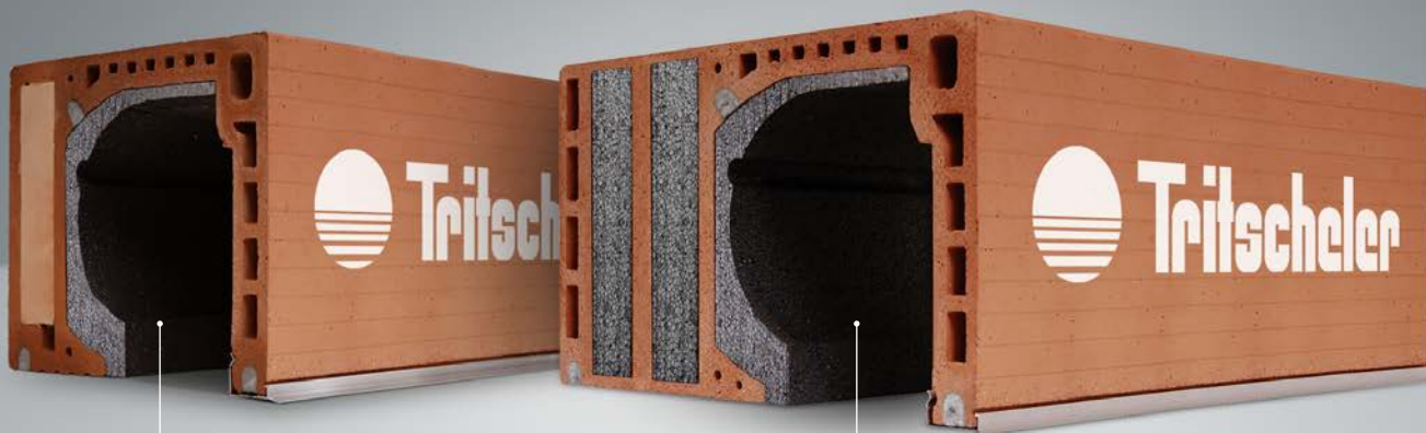
Ziegelkasten ThermoTon 38 für eine Wandstärke von 38 cm
